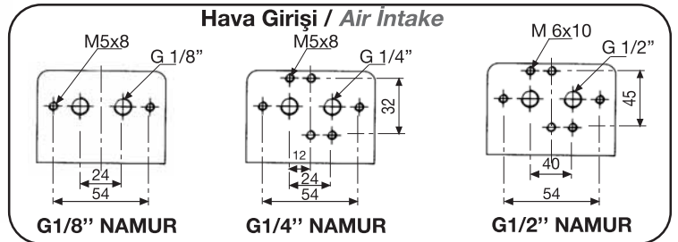
Tip-B Gövdeler / Type-B Body
